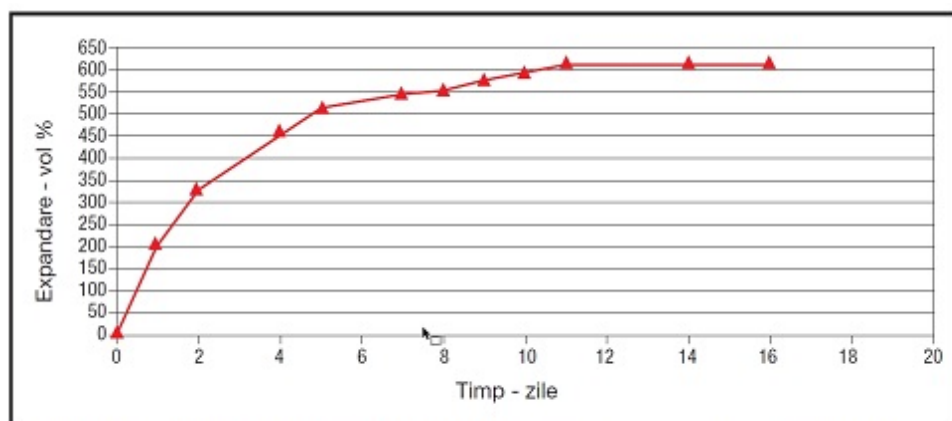
Fig. 1: graficul expandării volumetrice a Hidrostop Soft în apă distilată la +25°C în conformitate cu norma JIS K6258:1993
